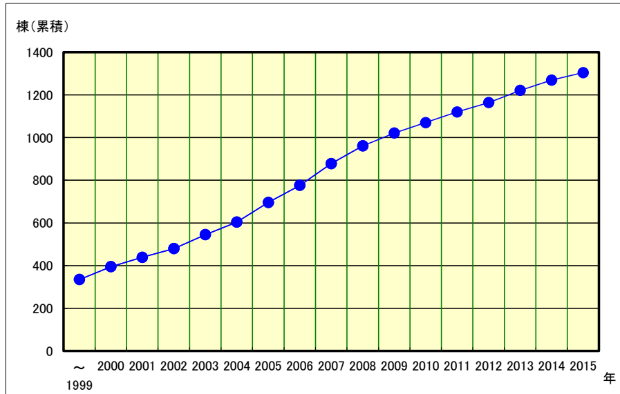
③制振建築物計画推移棟数(累積推移)
