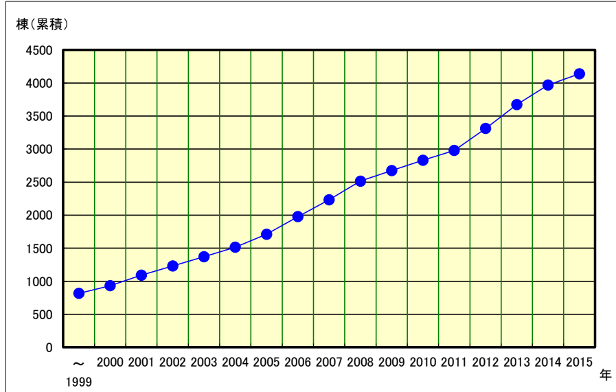
①免震建築物計画推移棟数(累積推移)
